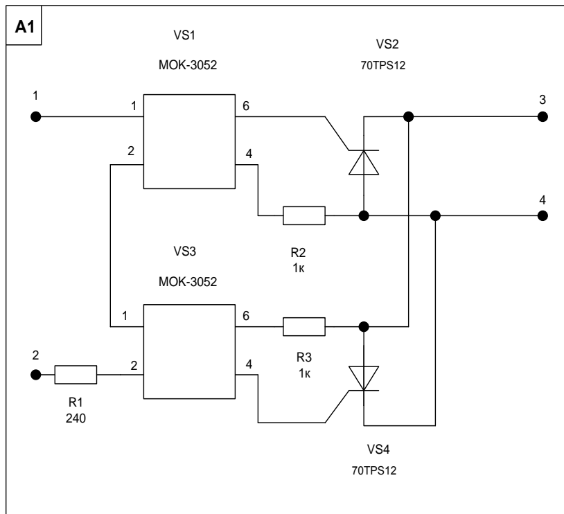
Рис. 1 Электролаборатория ЭТЛ-10. Блок управления. Плата А1. Тиристорный регулятор. Схема электрическая принципиальная
