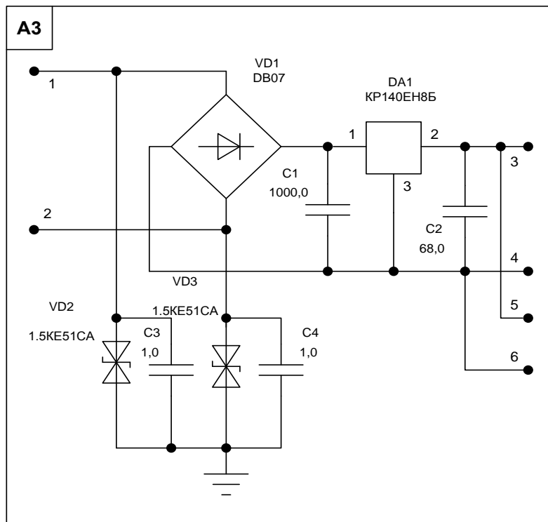
Рис. 2 Электролаборатория ЭТЛ-10. Блок управления. Плата А3. Стабилизатор напряжения. Схема электрическая принципиальная
